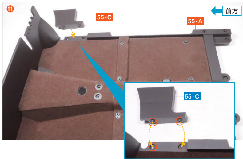
將前圍側裝飾板(R) 55-C 的兩個螺絲孔突起部分對準 55-A 的兩個螺絲孔凹槽插入。
