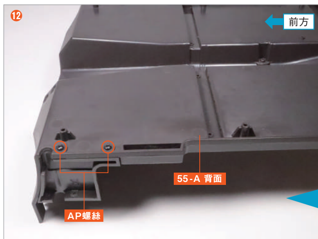
一邊按住 55-C 以防其脫落, 一邊將 55-A 翻過來, 並使用 AP 螺絲 固定兩處。
