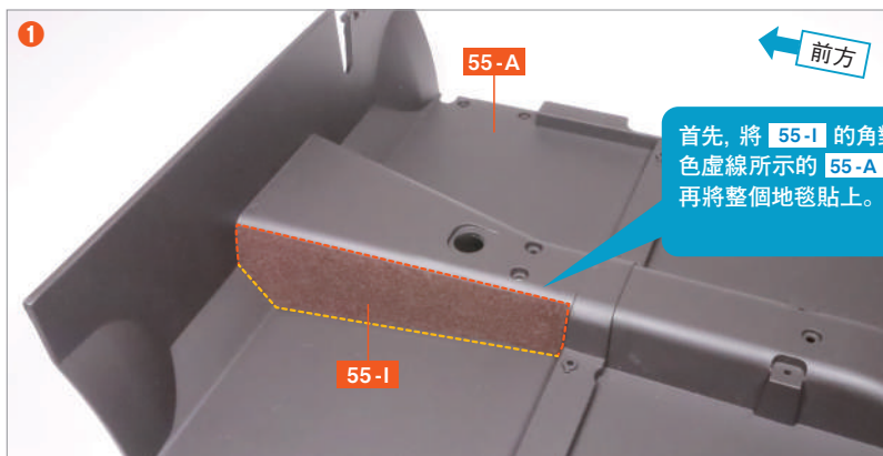
將中央地板地毯 (1) 55-I 從底紙上撕下，如照片所示貼在地板底板 55-A 上。
